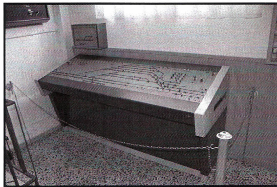
LA MESA NX DE REUS EN EL LOCAL SOCIAL
